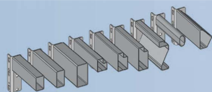
Feuillure 45x36 mm Feuillure 65x36 mm Feuillure 85x36 mm
